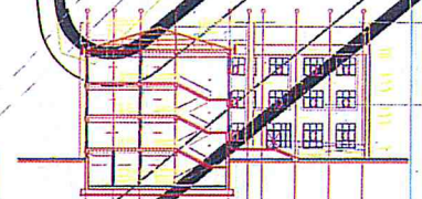
A-A KESİTİ ÖLÇEK : 1/200
